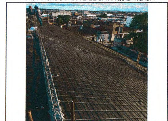
FORMA EM COMPENSADO PLÁSTIFICO E FERRAGENS DA LAJE DA ARQUIBANCADA
