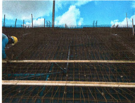
FORMA EM COMPENSADO PLÁSTIFICADO E FERRAGENS DA LAJE DA ARQUIBANCADA
