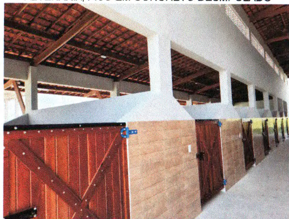
BAIAS COBERTAS - REVESTIMENTO CERÂMICO; PINTURA INTERNA; CANCELAS DE MADEIRA
