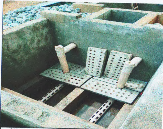
SISTEMA DE TRATAMENTO DE ESGOTO - FILTRO
