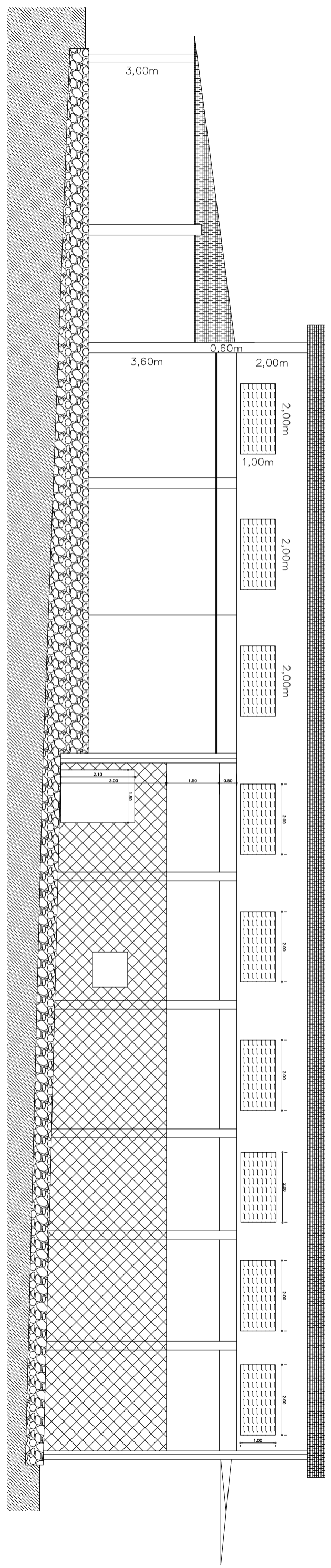
Corte B-B
