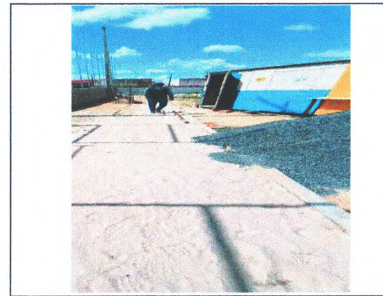
COLCHÃO DE AREIA PARA EXECUÇÃO DE PISO EM CONCRETO DESEMPOLADO.
