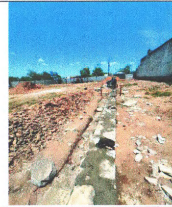
ESCAVAÇÃO E ALVENARIA DE PEDRA CONTENÇÃO QUADRA.
