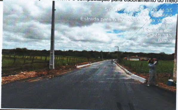
FOTO 12-Execução do aterro e compactação para escoramento do meio-fio
