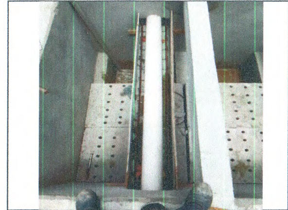
FILTRO - PLACAS E CALHA EM CONCRETO ARMADO
