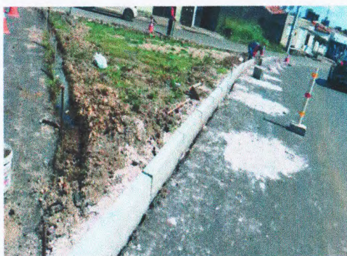
ASSENTAMENTO DE MEIO-FIO - ROTATÓRIA 01
