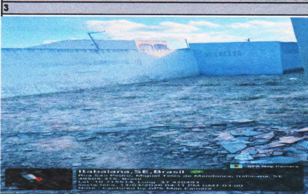
Imagem 3 - Demolição do piso de concreto simples
