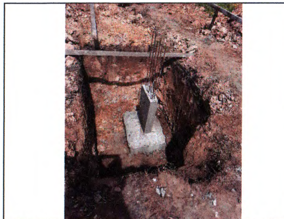
ESCAVAÇÃO; LOCAÇÃO COM GABARITO DE MADEIRA; CONCRETO ARMADO SAPATA E ARRAQUE DE PILAR
