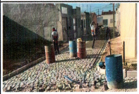
ASSENTAMENTO DE MEIO-FIO, DRENAGEM SUPERFICIAL E PAVIMENTAÇÃO - TRAVESSA PROJETA 04
