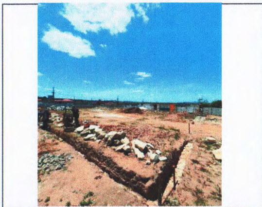
ESCAVAÇÃO E CONTENÇÃO EM ALVENARIA DE PEDRA.
