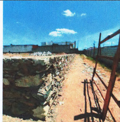
CONTENÇÃO EM ALVENARIA DE PEDRA.
