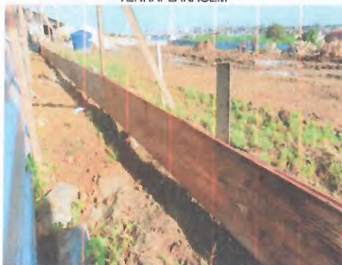
LOCAÇÃO DE OBRA: GABARITO
