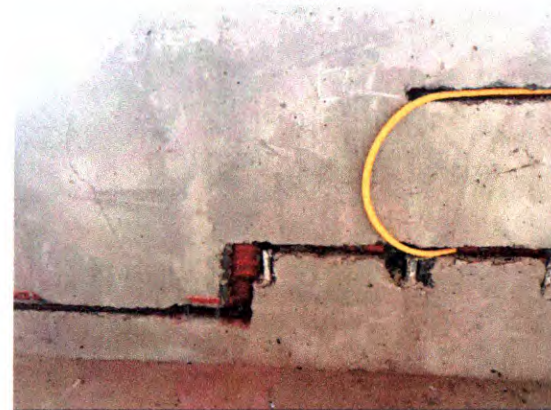
ALVENARIA DE BLOCO CERÂMICO; CHAPISCO; REBOCO; TUBULAÇÃO ÁGUA FRIA, ESGOTO E ELÉTRICA
