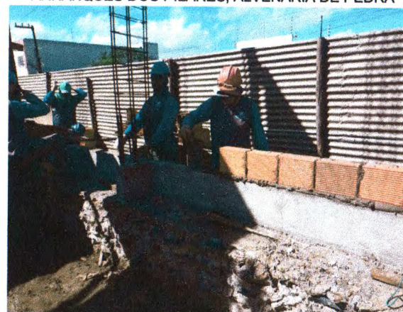
CONCRETO ARMADO PILARES E CINTA INFERIOR; ALVENARIA DE PEDRA ARGAMASSADA E BLOCO CERÂMICO; TAPUME METÁLICO
