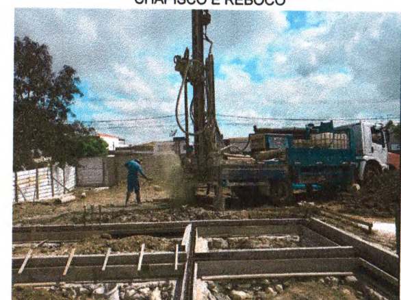
EXECUÇÃO DO ABRIGO DOS RESERVATÓRIOS PARA IRRIGAÇÃO; PERFURAÇÃO DO POÇO ARTESIANO
