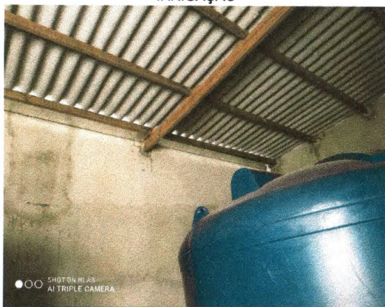
COBERTURA DO ABRIGO DOS RESERVATÓRIOS - MADEIRAMENTO E TELHAMENTO; CALHA EM ALUMÍNIO
