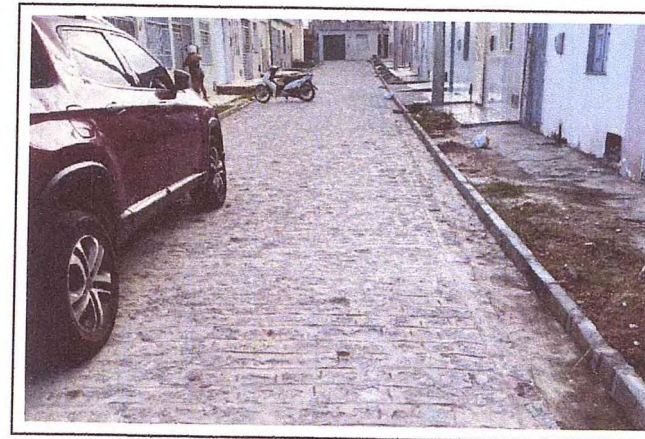
DRENAGEM SUPERFICIAL, PAVIMENTAÇÃO E ASSENTAMENTO DE MEIO FIO - TRAVESSA JOSÉ SIZINIO DE ALMEIDA 4
