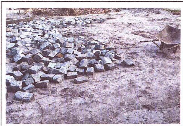
REGULARIZAÇÃO, ASSENTAMENTO DE MEIO-FIO, COLÇÃO DE AREIA - RUA JOSÉ PAULO VIEIRA
