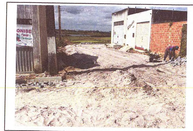
REGULARIZAÇÃO, COLCHÃO DE AREIA, ASSENTAMENTO DE MEIO-FIO - PROLONGAMENTO DA RUA JOSÉ SIZINIO DE ALMEIDA E VICE PREFEITO JOSIAS DA SILVA NUNES
