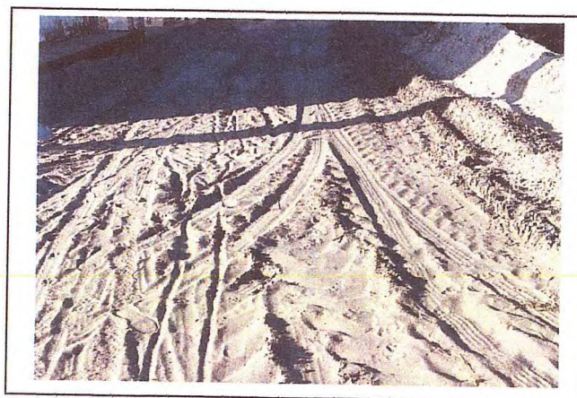
REGULARIZAÇÃO, COLCHÃO DE AREIA - PROLONGAMENTO DA RUA JOSÉ SIZINIO DE ALMEIDA E VICE PREFEITO JOSIAS DA SILVA NUNES
