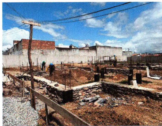
ALVENARIA DE PEDRA, VIGA BALDRAME E PINTURA ASFALTICA
