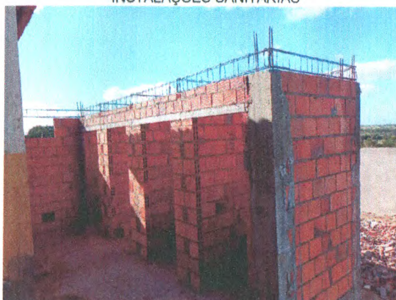
BANHEIROS NOVOS - CONCRETO ARMADO; ALVENARIA DE BLOCO CERÂMICO
