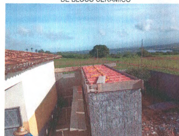
BANHEIROS NOVOS - CONCRETO ARMADO; ALVENARIA DE BLOCO CERÂMICO; CHAPISCO; LAJE PRÉ-MOLDADA
