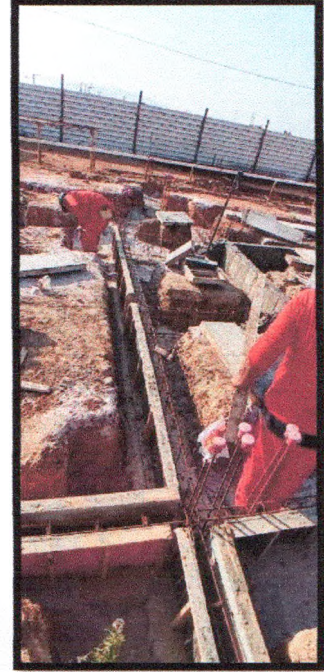
Figura 22: Concretagem de vigas baldrames
