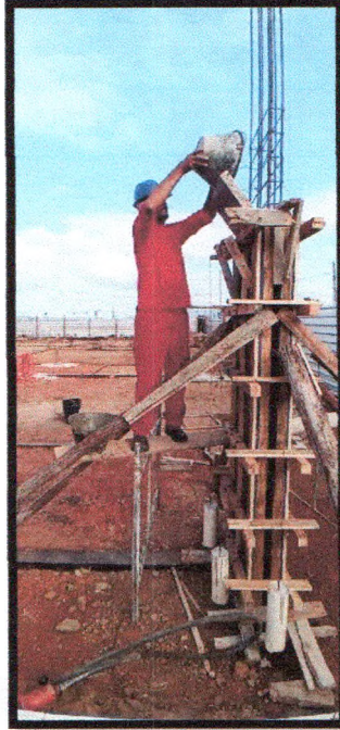
Figura 33: Montagem de forma para concretagem de pilar
