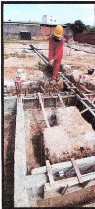
Figura 21: Concretagem de vigas baldrames
