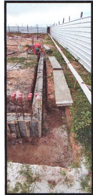
Figura 12: Concretagem de viga baldrame
