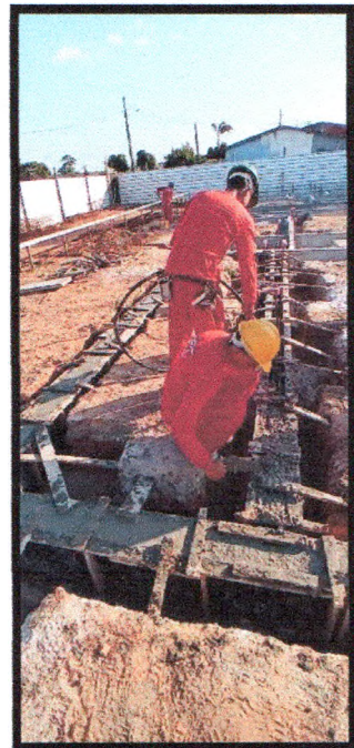
Figura 22: Concretagem de vigas baldrames
