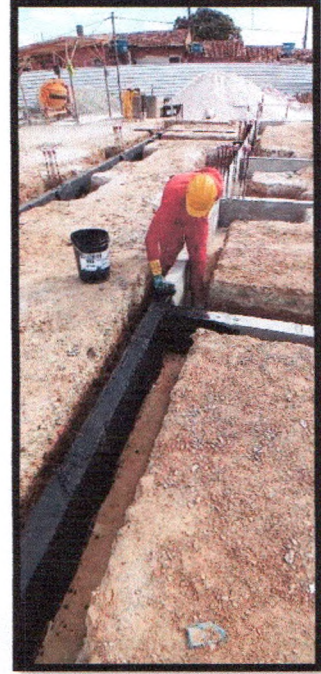
Figura 28: Impermeabilização das vigas baldrames
