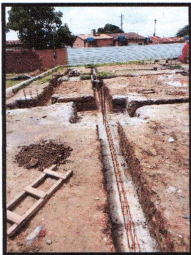
Figura 4: Execução de concreto magro das vigas baldrames
