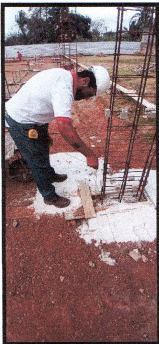
Figura 32: Colocação de armação para montagem de forma de pilar
