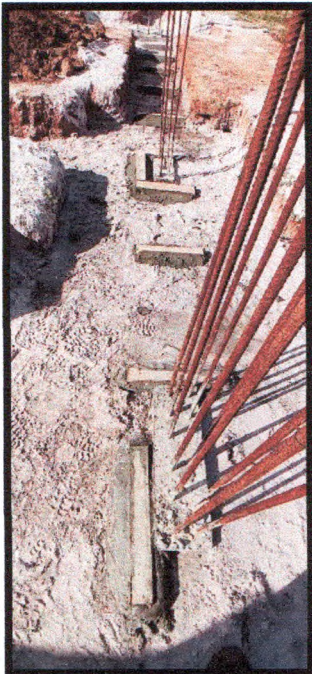
Figura 10: Execução de mestra para concreto magro de viga baldrame
