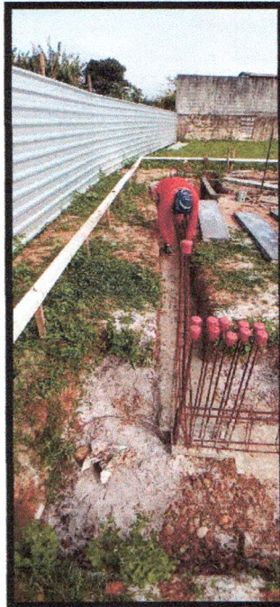
Figura 11: Execução de lastro de concreto magro de viga baldrame
