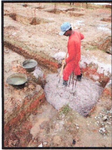
Figura 2: Execução de aterro e adensamento de cava de sapata
