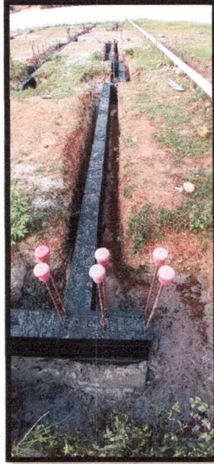
Figura 27: Impermeabilização das vigas baldrames
