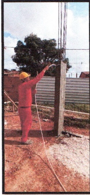
Figura 39: Retirada de forma de pilar concretado
