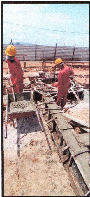
Figura 20: Concretagem de vigas baldrames
