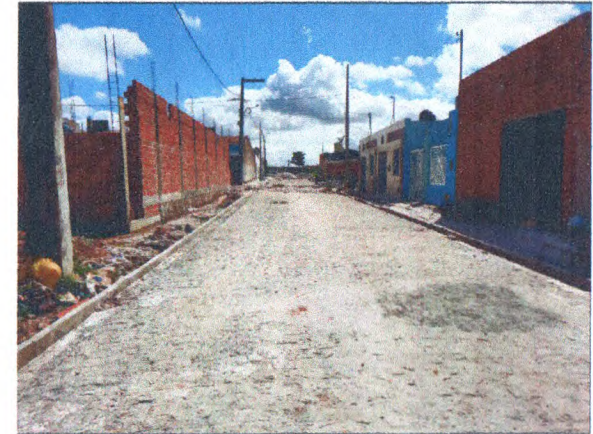
RUA JOSÉ VICENTE DE ALMEIDA - ASSENTAMENTO MEIO-FIO E PARALELEPÍPEDO; DRENAGEM SUPERFICIAL
