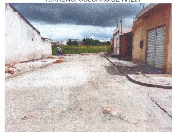
RUA JOSÉ ERALDO SANTOS - ASSENTAMENTO MEIO-FIO E PARALELEPÍPEDO; DRENAGEM SUPERFICIAL
