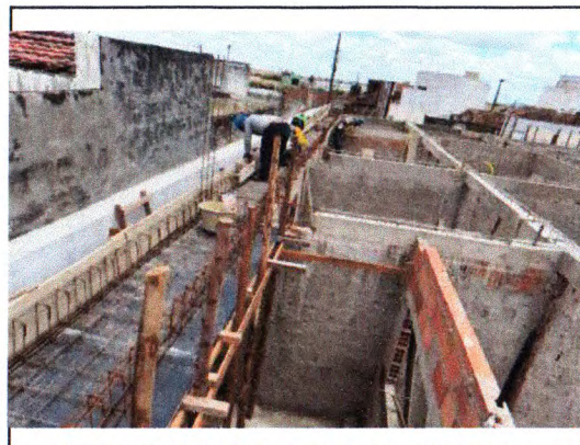
PREPARAÇÃO PARA LAJE MACIÇA
