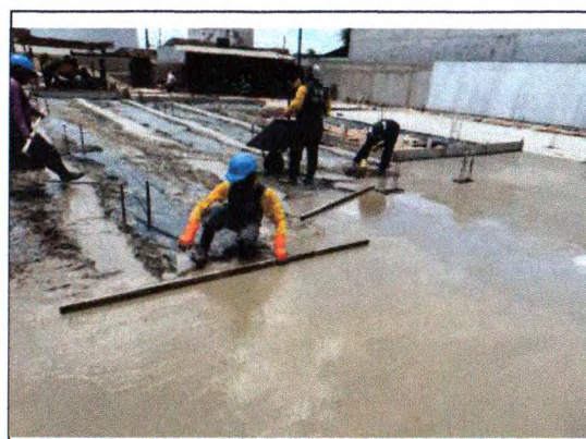
LONA PLÁSTICA E EXECUÇÃO DA CAMADA IMPERMEABILIZADORA
