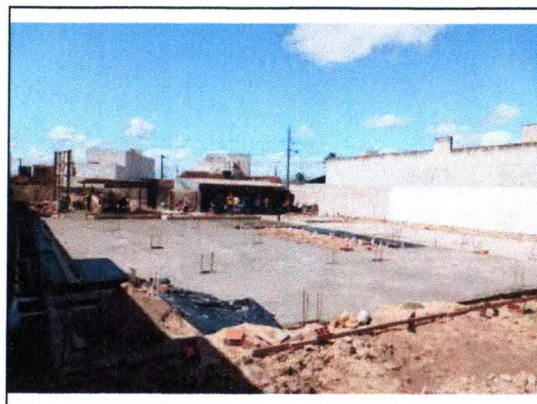
CAMADA IMPERMEABILIZADORA
