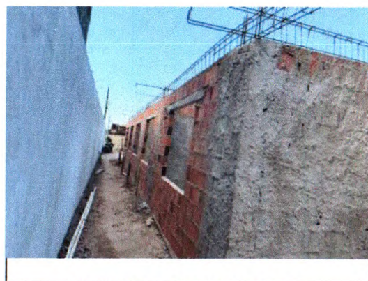
ELEVAÇÃO DE ALVENARIA, VIGAS, VERGAS, CONTAVERGAS E PLARES
