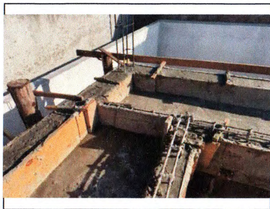
LAJE MACIÇA E VIGAS SUPERIORES
