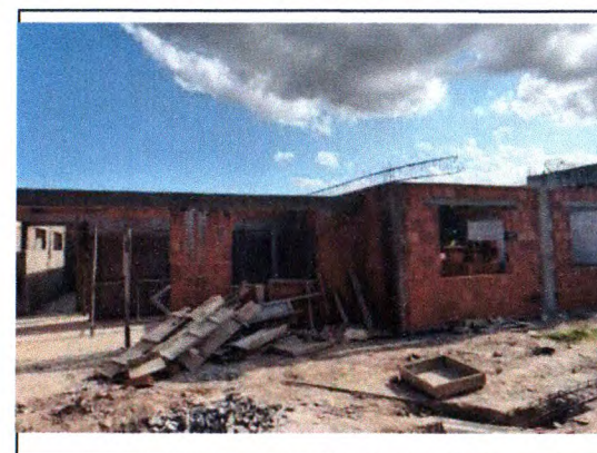
ELEVAÇÃO DE ALVENARIA, VIGAS, VERGAS, CONTAVERGAS E PLARES
