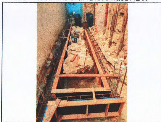
ESCAVAÇÃO; CONCRETO MAGRO; FORMA; FERRAGEM VIGAS E ARRANQUE PILAR
