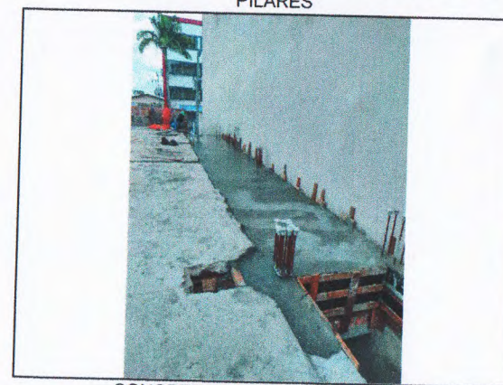
CONCRETAGEM DE VIGAS E LAJE
