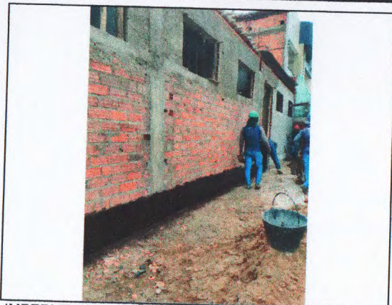
IMPERMEABILIZAÇÃO DE ESTRUTURA; ALVENARIA DE BLOCO; CHAPISCO, REBOCO
