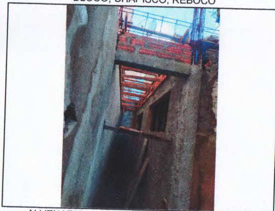
ALVENARIA DE BLOCO; CHAPISCO, REBOCO; FERRAGEM DE VIGAS E PILARES
