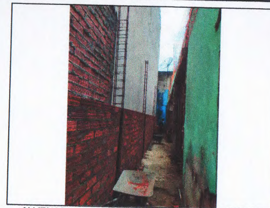
ALVENARIA DE BLOCO CERÂMICO; FERRAGEM DE PILARES
