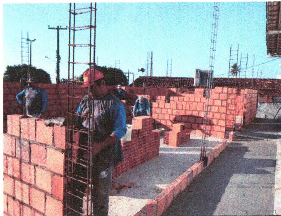
ALVENARIA DE BLOCO CERÂMICO; FERRAGEM DOS PILARES
