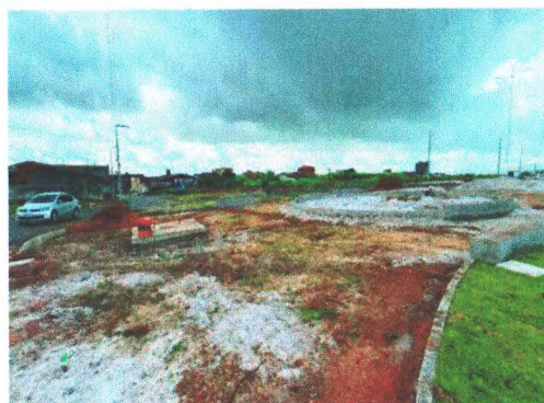
MEIO-FIO E EXECUÇÃO DE ATERRO DA ROTATÓRIA 01
