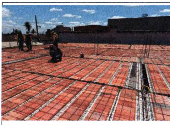
LAJE PRÉ MOLDADA
