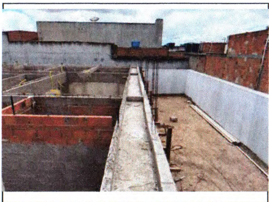
LAJE MACIÇA E VIGAS SUPERIORES
