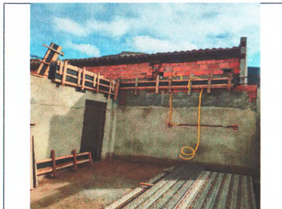
ALVENARIA DE BLOCO; CHAPISCO; REBOCO; VERGAS; CONCRETO ARMADO DE VIGAS
