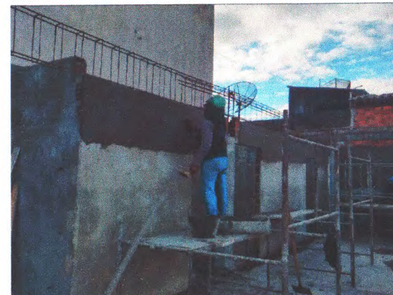
ALVENARIA DE BLOCO; CHAPISCO; REBOCO; VIGA EM CONCRETO ARMADO;
