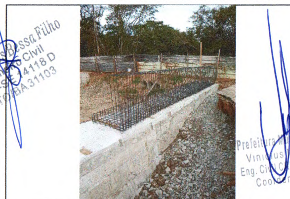
MONTAGEM DE AÇO DO BERÇO E CORTINA
