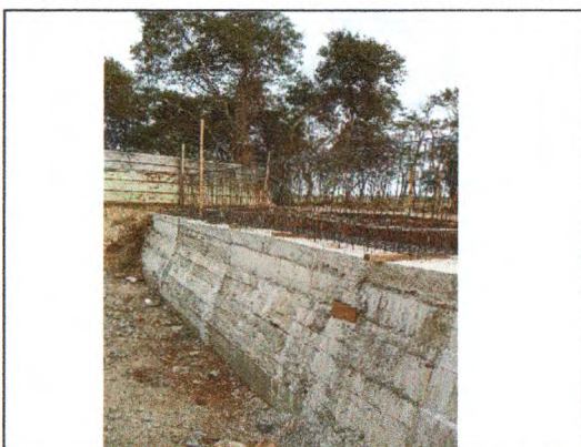
MONTAGEM DE AÇO DO BERÇO E CORTINA
