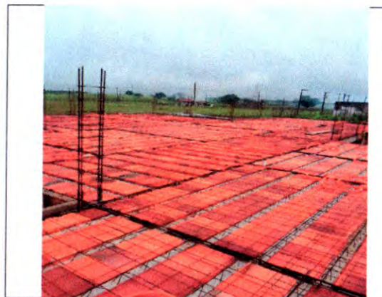
LAJE PRÉ MOLDADA
