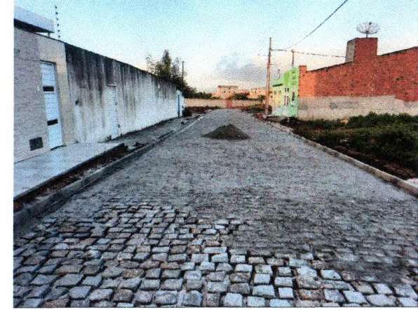
RUA PROJETADA "A" - ASSENTAMENTO MEIO-FIO E PARALELEPÍPEDO; DRENAGEM SUPERFICIAL
