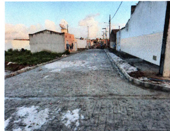
RUA JOSÉ VINCENTE DE ALMEIDA - REGULARIZAÇÃO DO TERRENO; COLCHÃO DE AREIA
