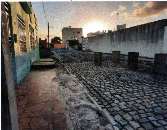
RUA PROJETADA "A" - ASSENTAMENTO MEIO-FIO E PARALELEPÍPEDO; DRENAGEM SUPERFICIAL
