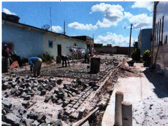
RUA FRANCISCA XAVIER NUNES - COLCHÃO DE AREIA; ASSENTAMENTO MEIO-FIO E PARALELEPÍEDO; DRENAGEM SUPERFICIAL
