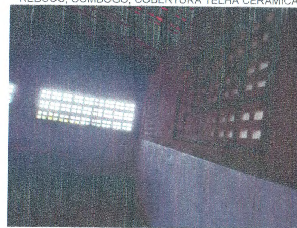
AMPLIAÇÃO - ALVENARIA DE BLOCO; CHAPISCO; REBOCO; COMBOGÓ; COBERTURA TELHA CERÂMICA; REVESTIMENTO CERÂMICO; REGULARIZAÇÃO DO PISO
