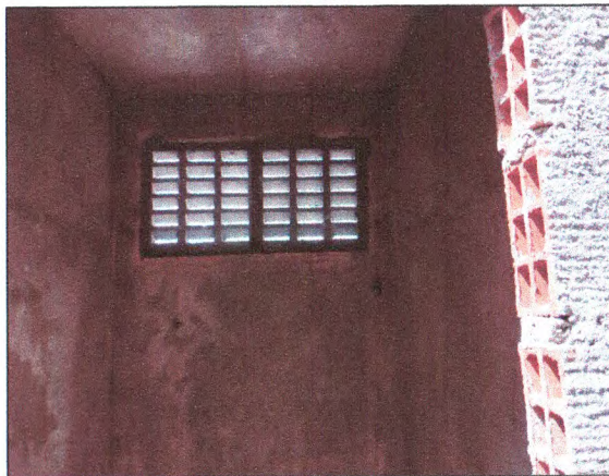
BANHEIRO - ALVENARIA DE BLOCO CERÂMICO; CHAPISCO; REBOCO; COMBOGÓ DE CIMENTO
