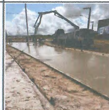
PISO EM CONCRETO COM LONA PLASTICA
