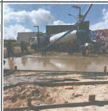
PISO EM CONCRETO COM LONA PLASTICA
