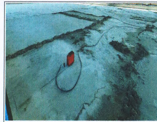
PISO DE ALTA RESISTÊNCIA - EXECUÇÃO
