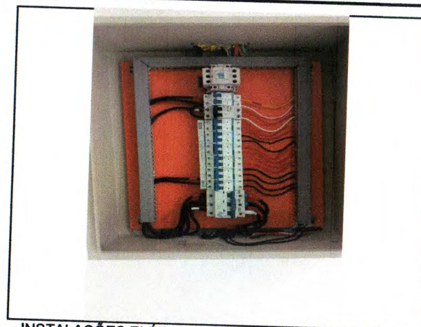
INSTALAÇÕES ELÉTRICAS - QUADRO, DISJUNTORES, CABOS E FIOS
