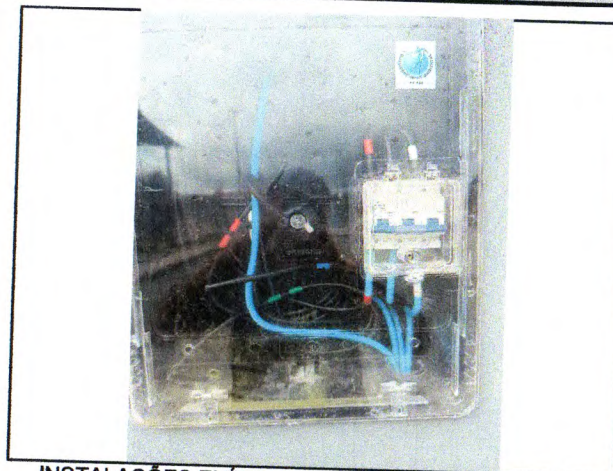
INSTALAÇÕES ELÉTRICAS - QUADRO DE MEDIÇÃO; DISJUNTOR E CABOS
