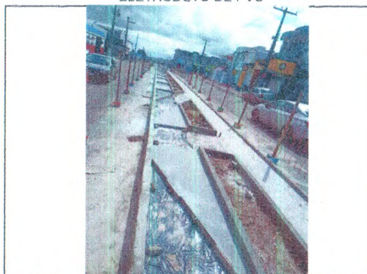
TAPUME DE PROTEÇÃO EM TELA; MEIO-FIO EM CONCRETO; ATERRO COMPACTADO; LONA PLÁSTICA; PISO EM CONCRETO DESEMPOLADO
