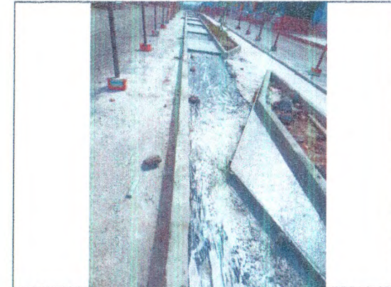
MEIO-FIO EM CONCRETO; ATERRO COMPACTADO; LONA PLÁSTICA; PISO EM CONCRETO DESEMPOLADO
