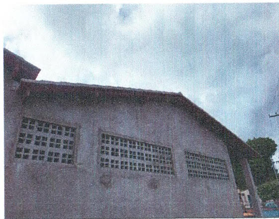
REVISÃO DA COBERTURA EM TELHA CERÂMICA; EMASSAMENTO DE BEIRAL
