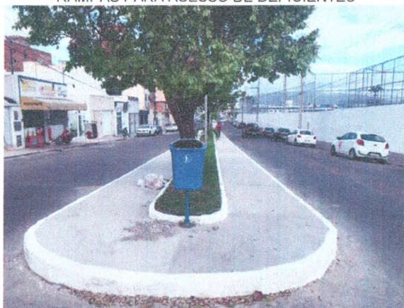
PISO EM CONCRETO DESEMPOLADO; PINTURA MEIO-FIO; LIXEIRA; GRAMA ESMERALDA
