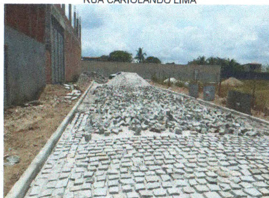
COLCHÃO DE AREIA, MEIO FIO E PARALELEPIPEDO NA TRV. PROJETADA 02
