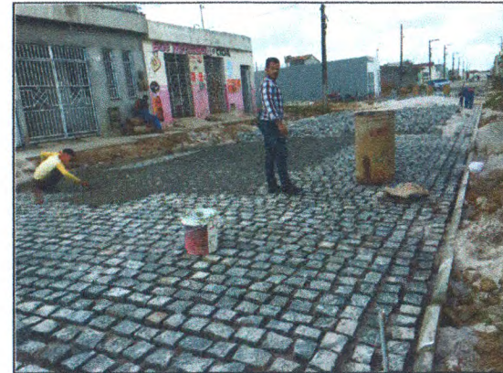
PAVIMENTAÇÃO NA RUA JOSIVAL NUNES DOS SANTOS
