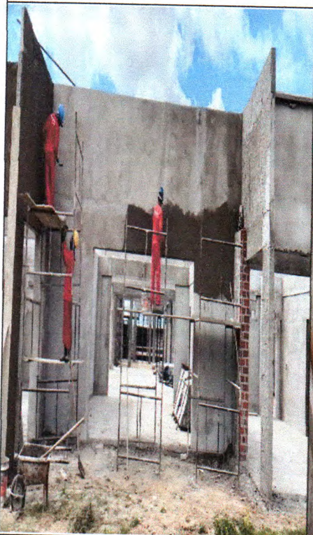
Figura 11 : Reboco ou emboço externo, de parede
