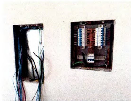
INSTALAÇÕES ELÉTRICAS
