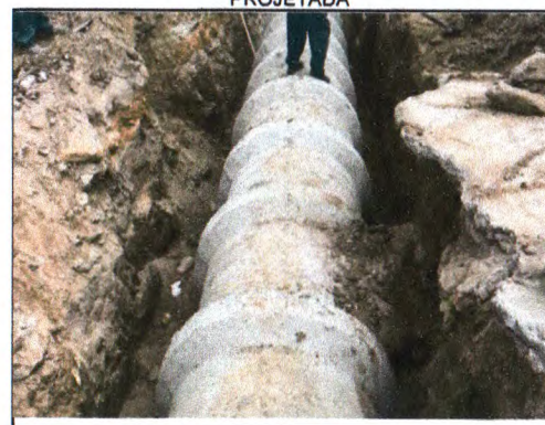
DRENAGEM PROFUNDA - TUBULAÇÃO CENTRAL
