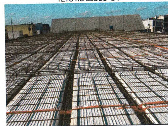
EXECUÇÃO DA LAJE DO BLOCO C;
