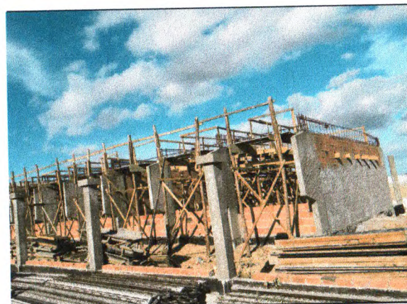
EXECUÇÃO DA ALVENARIA DE BLOCO CERÂMICO; CHAPISCO; REBOCO NO BLOCO "C";
