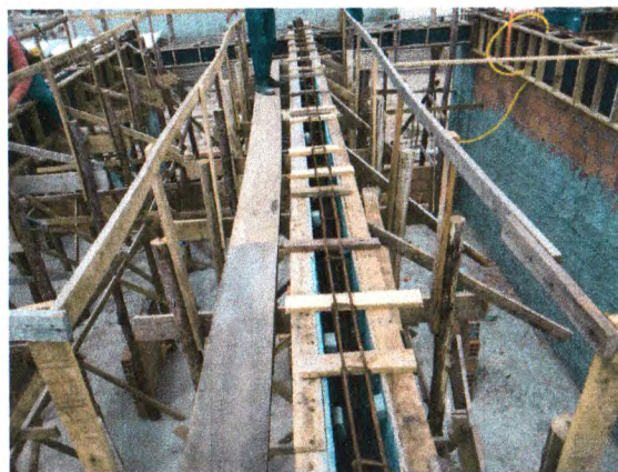
EXECUÇÃO DAS VIGAS DO BLOCO C - ESCORAMENTO, FORMA E FERRAGEM;
