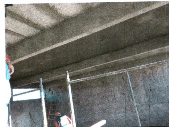
EXECUÇÃO DO CHAPISCO E REBOCO DE PAREDES E TETO NO BLOCO "B";
