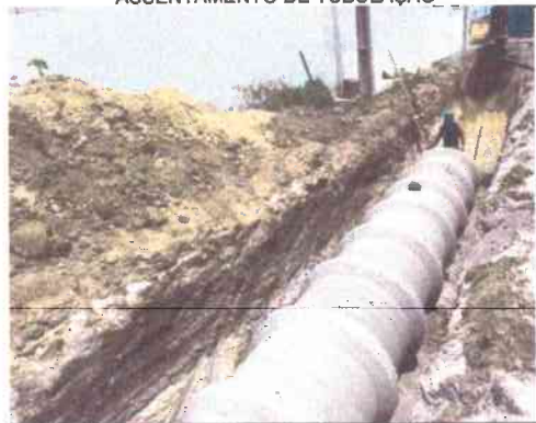
DRENAGEM PROFUNDA - ESCAVAÇÃO E ASSENTAMENTO DE TUBULAÇÃO
