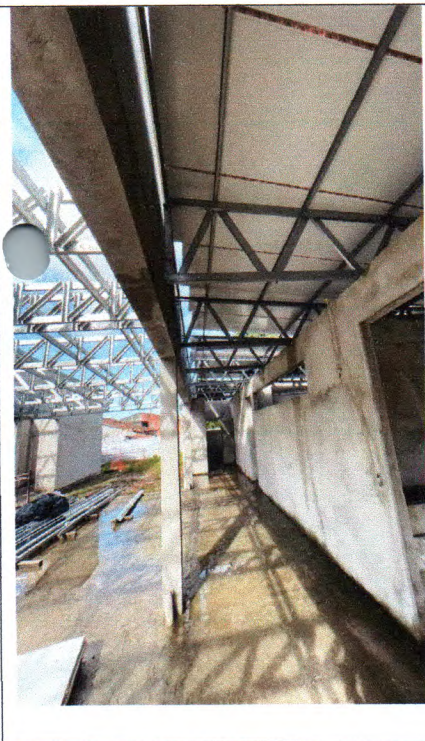
Figura 16: Telhamento com telha em aço galvanizado, dupla trapezoidal, na etapa B
