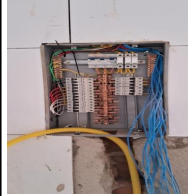
INSTALAÇÕES ELÉTRICAS
