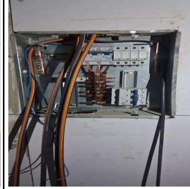
INSTALAÇÕES ELÉTRICAS
