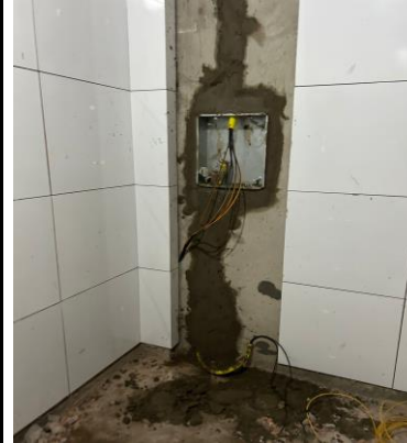
INSTALAÇÕES ELÉTRICAS
