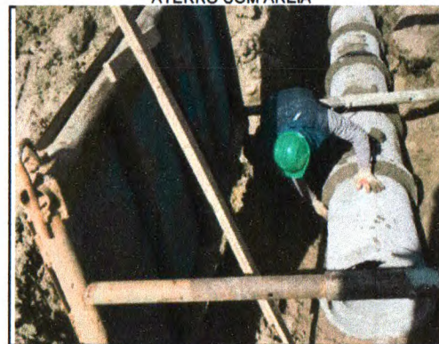
DRENAGEM PROFUNDA - ESCORAMENTO METÁLICO
