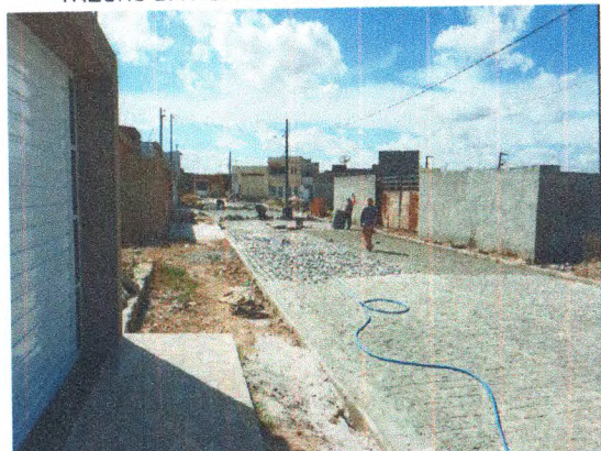
MEIO FIO E PARALELEPIPEDO TRECHO DA RUA TERCILIA PASSOS OLIVEIRA
