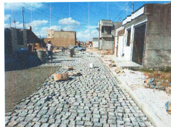
COLCHÃO DE AREIA, MEIO FIO E PARALELEPIPEDO NA RUA ANTÔNIO OLIVEIRA
