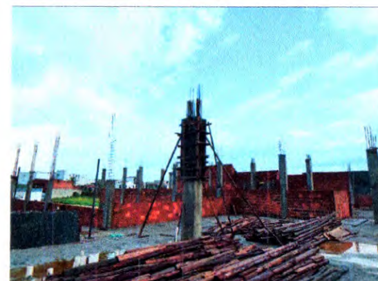
ALVENARIA DE VEDAÇÃO, FORMA E CONCRETO DOS PILARES
