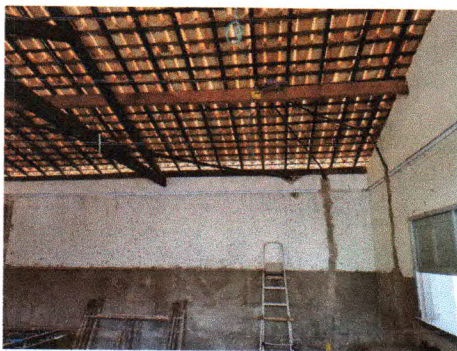
Fotos 05. Apicotamento de paredes; execução de reboco; substituição de eletrodutos e caixas de passagens; instalação de cabeamento elétrico. Instalação de saboneteiras
