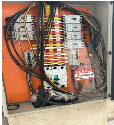
INSTALAÇÕES ELÉTRICAS: CABOS E DISJUNTORES
